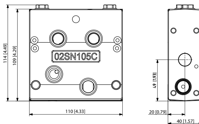
PVB 16 dimensions
